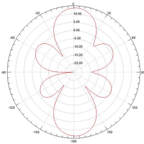
垂直面方向图
