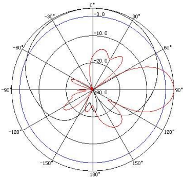
辐射方向图
