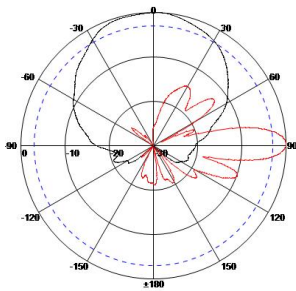
方向图
