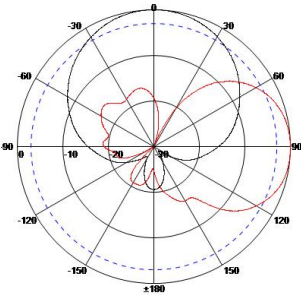
698-960MHz 频段方向图
