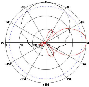
1710-2690&3300-3700MHz 频段方向图
