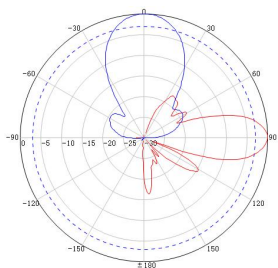
1710-2690MHz 频段方向图
