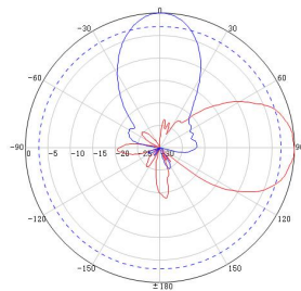
703-960MHz 频段方向图
