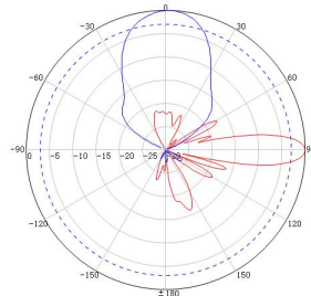
3300-3800MHz 频段方向图
