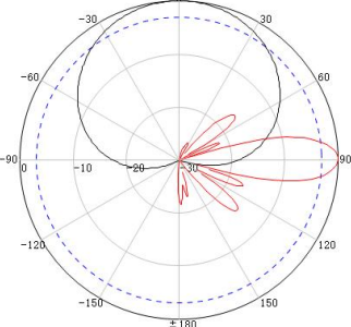
3300-3800MHz 频段方向图
