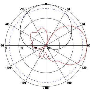
750-960MHz 频段方向图
