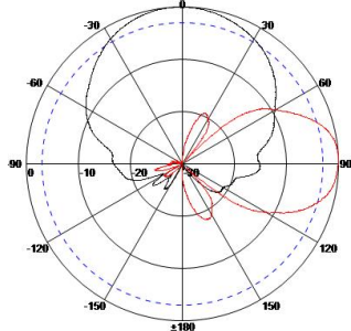
1710-2690MHz 频段方向图
