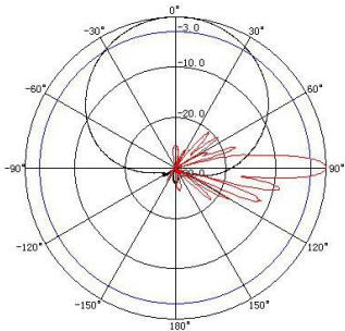
辐射方向图
