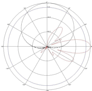
辐射方向图
