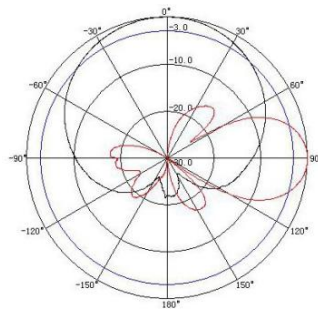
辐射方向图
