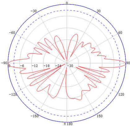
方向图
