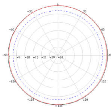
水平面方向图
