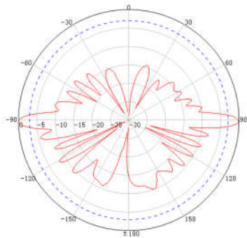
垂直面方向图
